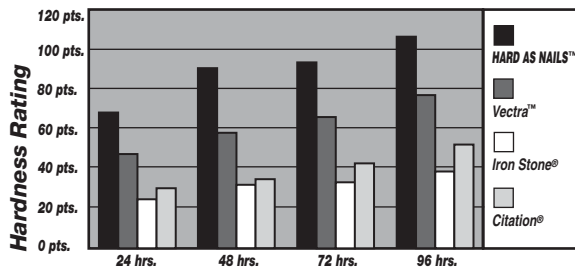
Koenig Pendulum Hardness Tester*
